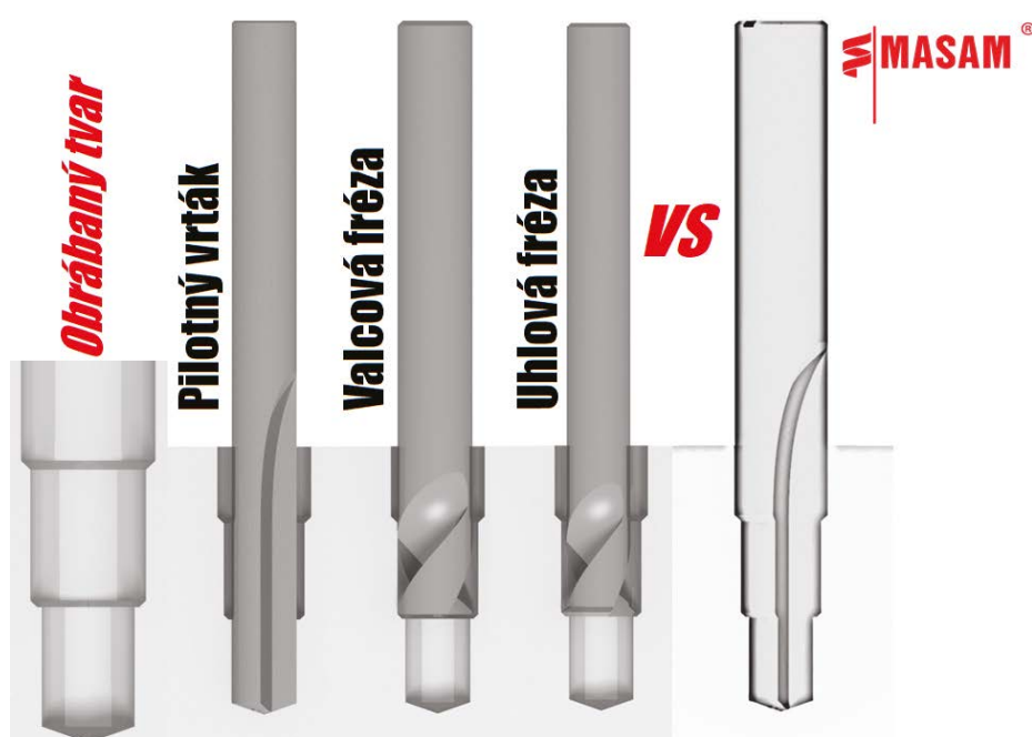
Príklad výroby stupňovitého otvoru
