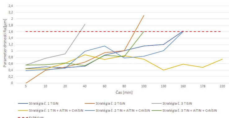
Porovnanie trvanlivosti povlakov pre kritérium Ra
